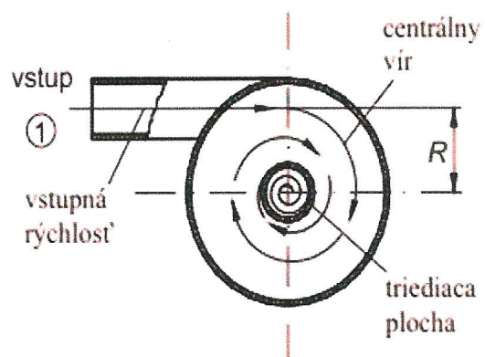
Obr. 1: Schéma hydrocyklón
